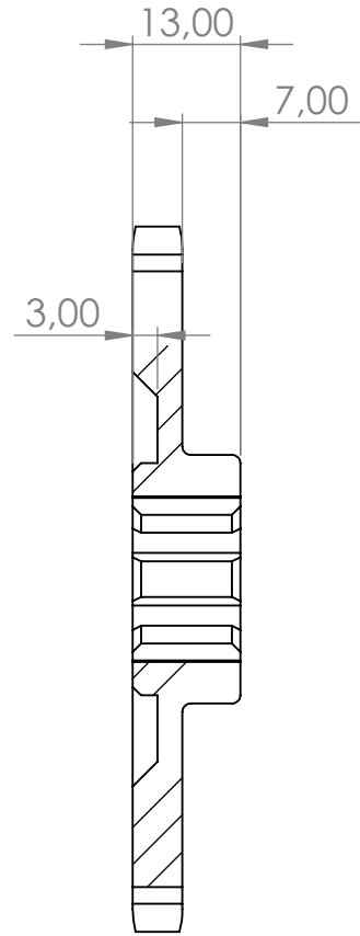
SEZIONE A-A
