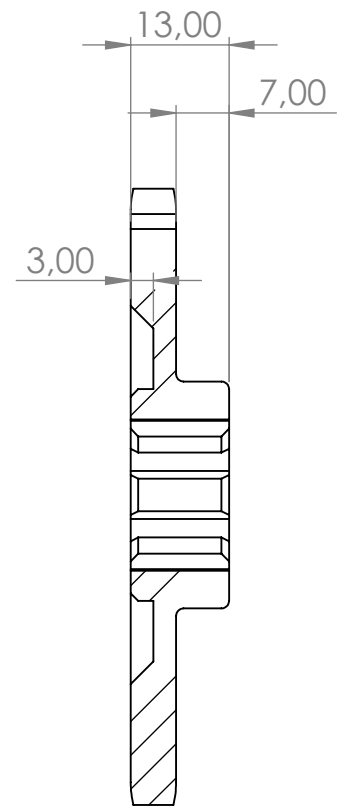
SEZIONE A-A
