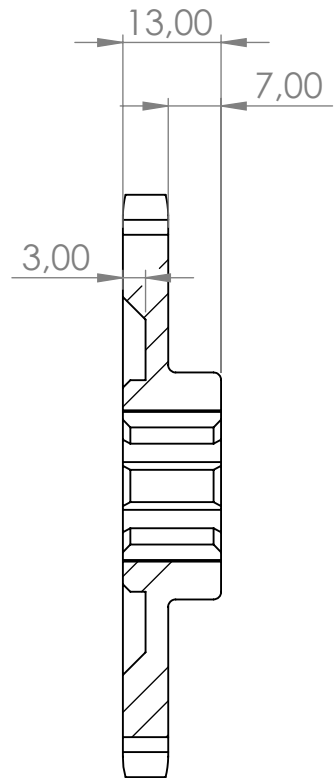
SEZIONE A-A
