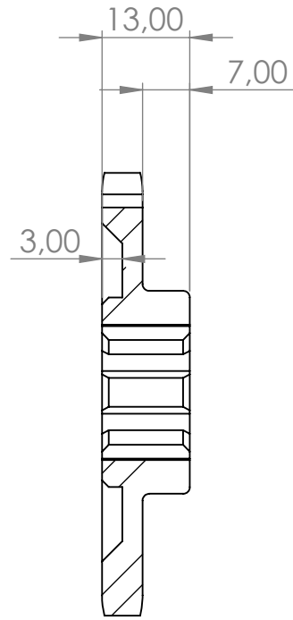
SEZIONE A-A
