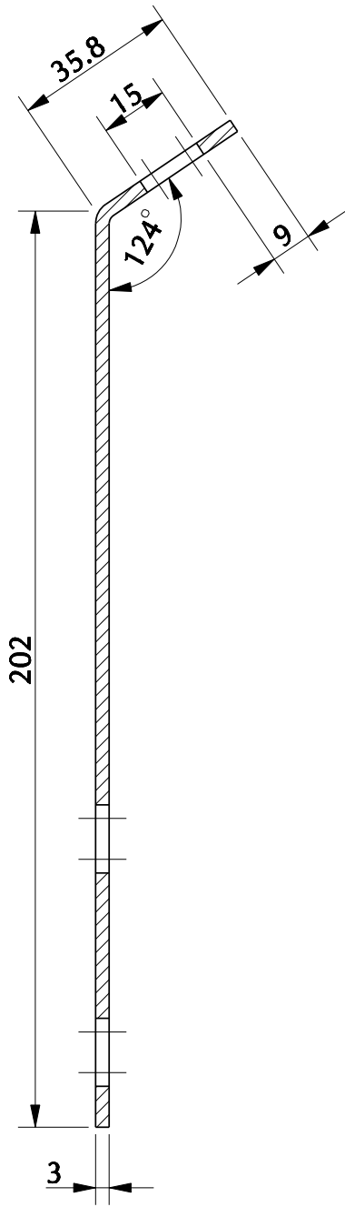
SEZIONE A-A
